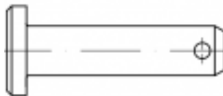
Sworznie z łbem walcowym DIN 1434, 1444, 1435,1436/ PN-83002/ ISO 2341
