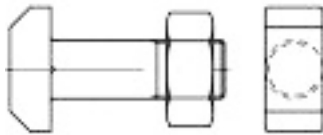
Śruby z łbem młoteczkowym DIN 261/ PN- 82424
