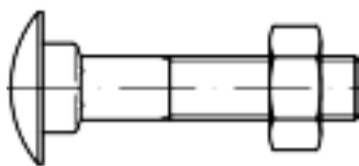
Śruby z łbem grzybkowym z podsadzeniem kwadratowym (zamkowe) DIN 603/ PN-82406/ ISO 8677
