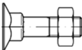
Śruby z łbem stożkowym z podsadzeniem kwadratowym (płużne) DIN 605 i DIN 608/ PN-82402
