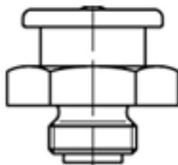
Smarowniczki ciśnieniowe kulkowe z główką prostą DIN 3404
