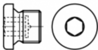
Korki gwintowane z kołnierzem i gniazdem sześciokątnym DIN 908
